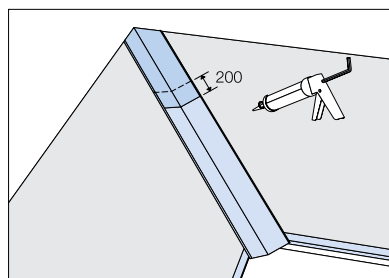
A vápalemez szegélylemezek hosszirányú átfedése legalább 200 mm legyen. Az átfedésben használjunk tartósan rugalmas, vízzáró tömítést.
