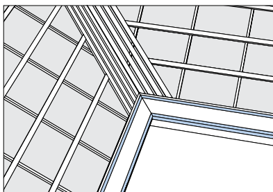
Lécekre történő szereléskor a vápa aljzatának felső síkja essen egybe a lécezés felső síkjával.
