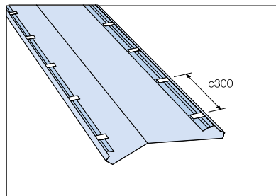
Helyezzük a C2SRP beakasztó rögzítőlemezeket a vápalemez felfordított széleihez mindkét oldalon. Vágjunk ki 30 mm-es fércet egy rögzítőlemezről, és helyezzük el ezeket egymástól 300 mm-nyire a széle mentén.
