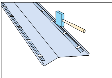
Rögzítsük a rögzítő lemezt a vápalemez szegélylemez élének lekalapálásával.
