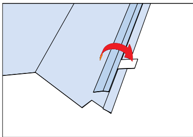
Hajlítsuk fel a férclemezeket az élen keresztül. Ezek lesznek a vápalemez tetőhöz való rögzítési pontjai.
