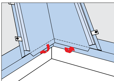
Hajlítsuk be a vápalemez alsó, túlnyúló végét a beakasztó ereszszelegélyhez rögzítve.
