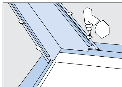
Helyezzük a vápalemezt a pontos helyére, és rögzítsük csavarokkal a férclemezekon keresztül.
